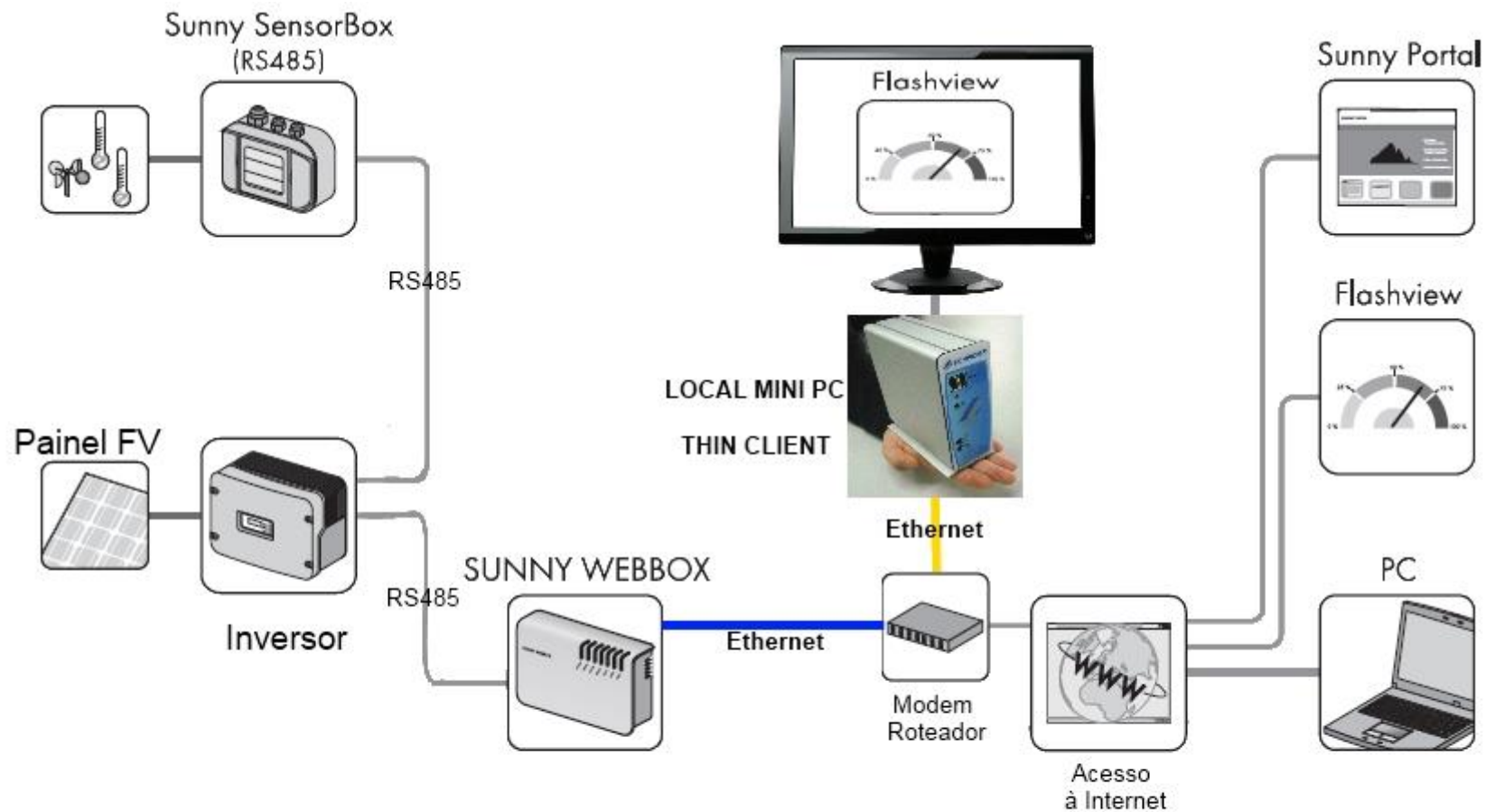
DIAGRAMA SIMPLIFICADO DE INTERCONEXÃO DOS COMPONENTES
